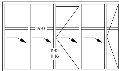
HSW mit Dreh-Schiebeflügel und Sprosse HSW with Incorporated Pass Door and transom rail
