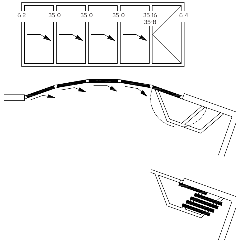
segmentierter Grundriss segmented layout
