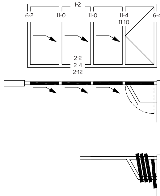
gerader Grundriss straight layout
