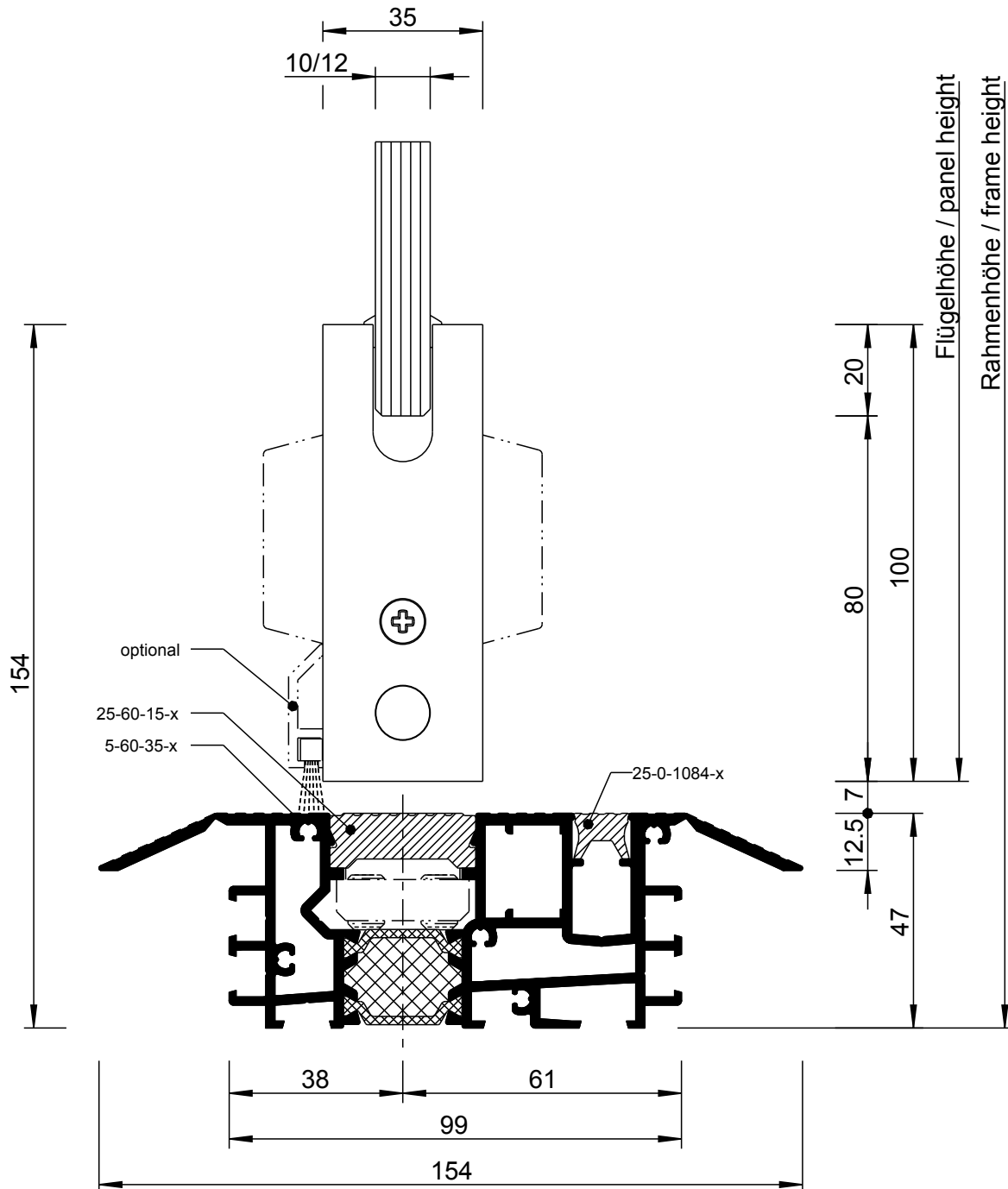
Detail GGHSW-2-12
